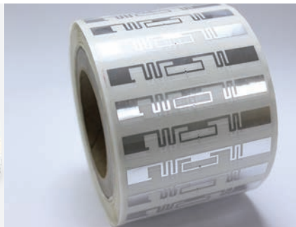
Étiquettes RFID UHF
